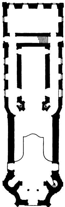
San Francisco en Ouro Preto (Alcapedrinho, 1766-94): Alzado y Planta.
